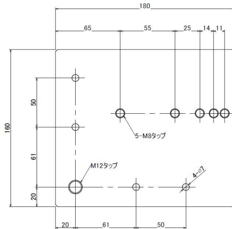
板厚t=6
