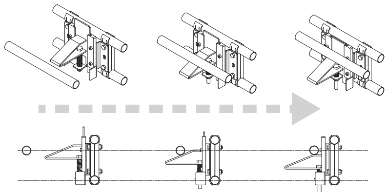
ストッパー解除イメージ
