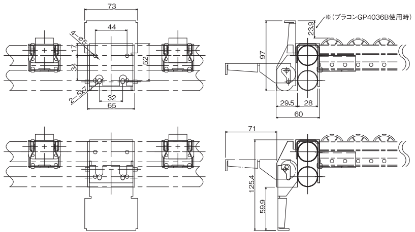
ストッパー解除イメージ
