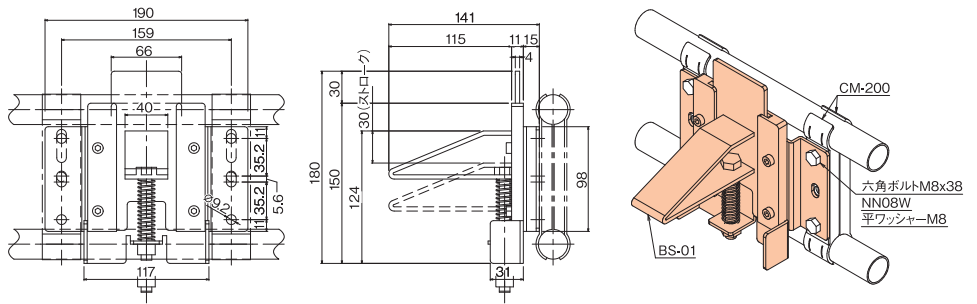
ストッパー解除イメージ
